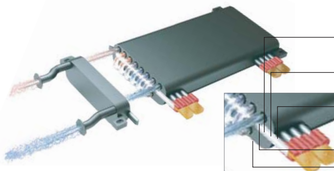
Внутренний вид котла Nobby Electro KBL
