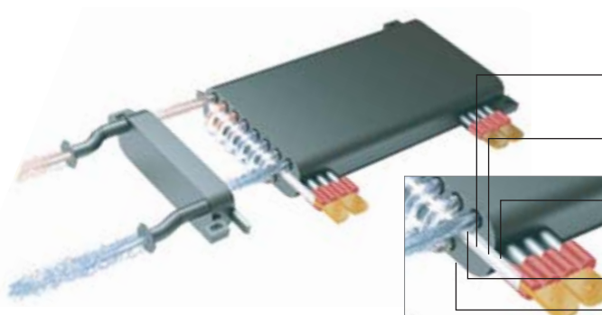
Внутренний вид котла Nobby Electro KBC
