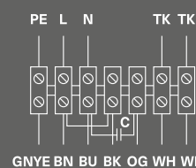
Схема 3 (400 В, 3 ф, 50 Гц.)
