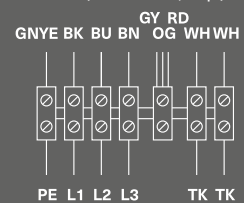
Схема 4 (λ — 400 В, 3 ф.)
