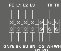
Схема 4 (λ — 400 В, 3 ф.)
