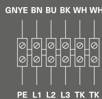
Схема 3 (400 В, 3 ф, 50 Гц.)
