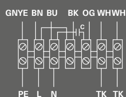
Схема 2 (230 В, 1 ф.)
