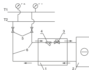
Возможная схема обвязки с 2-ходовым регулирующим клапаном
