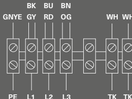
Схема 2 (400 В, 3 ф, 50 Гц.)
