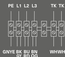
Схема 4 (Δ — 230 В, 3 ф.)
