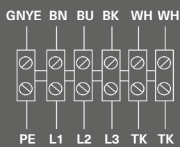
Схема 5 (400 В, 3 ф.)
